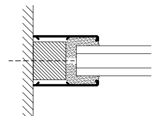
Wandanschluss
